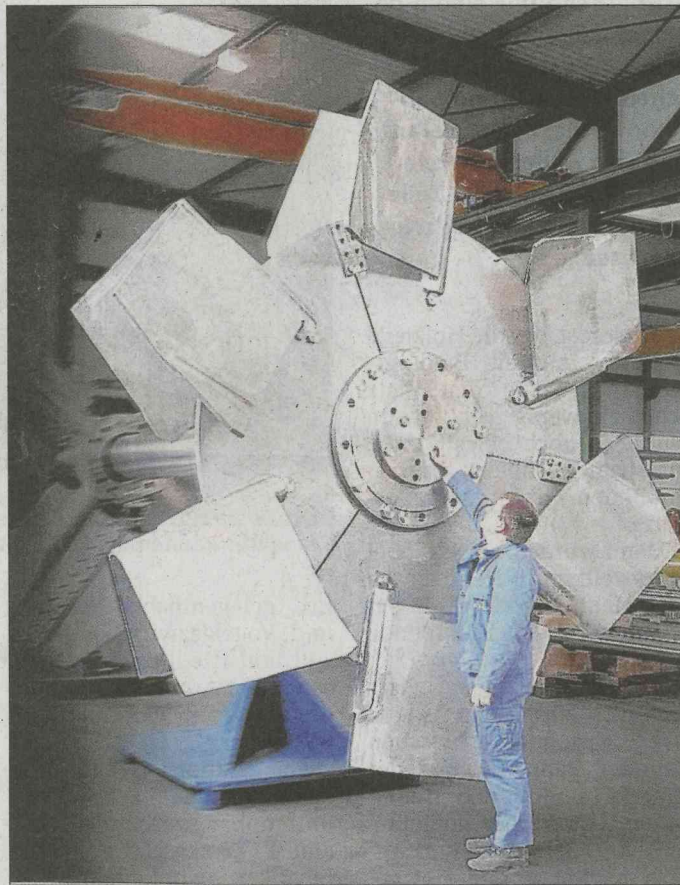
Die auf dem Markt gefragten, hochwertigen Titanrührwerke stellt die Ekato-Gruppe mit speziell ausgebildeten Fachkräften ausschließlich in Schopfheim her. Fotos: Ekato
